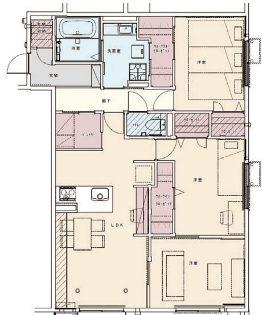
プランD 82.72㎡ 計3戸 家賃 62,000～64,000 円
