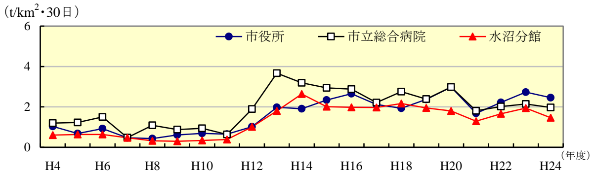
図4-4 降下ばいじん量の年平均値の経年変化
