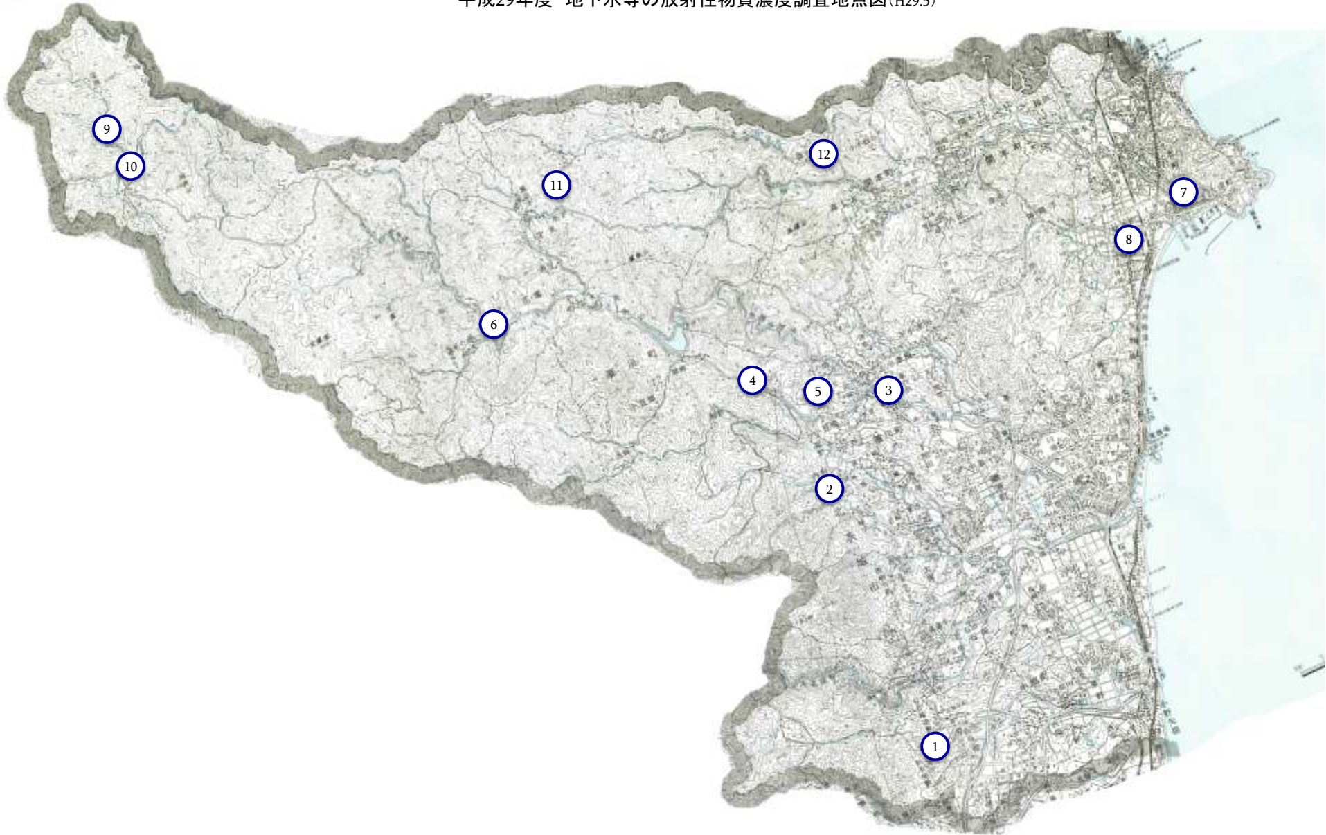
平成29年度 地下水等の放射性物質濃度調査地点図(H29.5)
