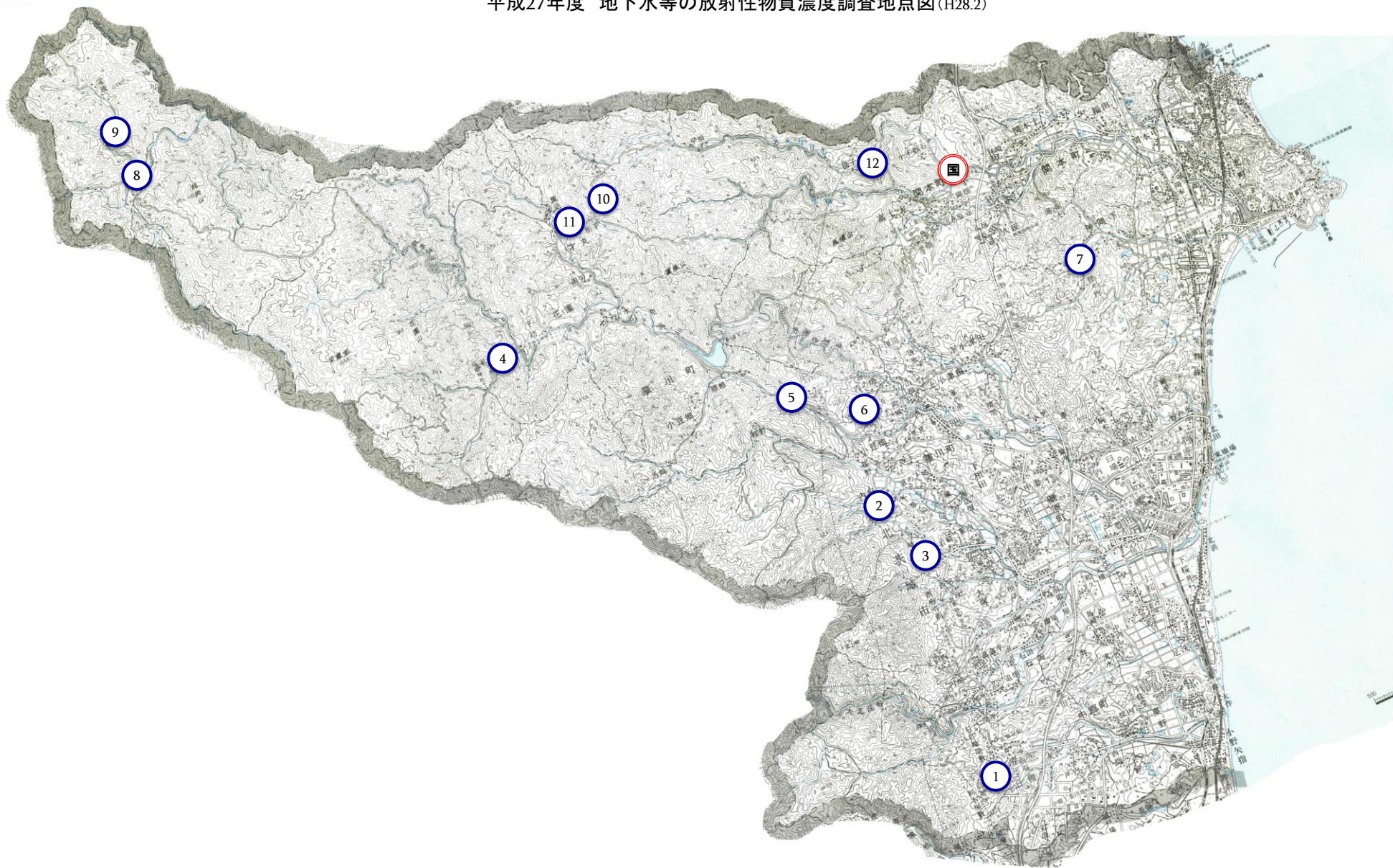
平成27年度 地下水等の放射性物質濃度調査地点図 (H28.2)
